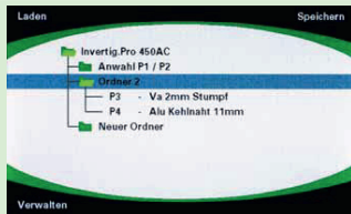
1. Programmordner
