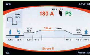
3. Programm laden
