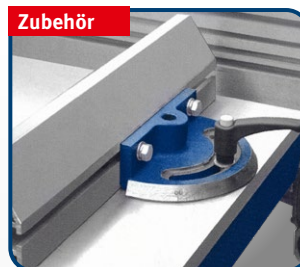
Gehrungsanschlag für KSO Art.-Nr.: 5379050
