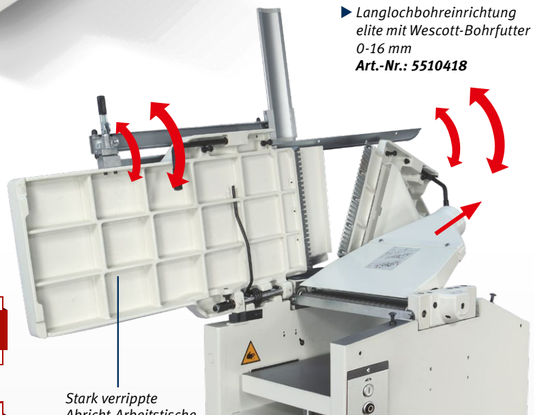
minimax fs 41e mit geöffneten Abrichtischen
