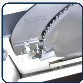
► Mikrodosiereneinrichtung direkt am Sägeblatt
