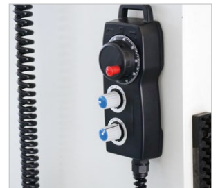
▶ Präzise Steuerung der Feinpositionierung über drei Drehknöpfe: oberer Knopf für die Positionierung, mittlerer zur Auswahl der Achse und unterer zur Einstellung der Schrittweiten 1, 10 oder 100
