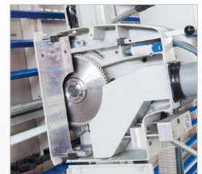
▶ Große Öffnung für Sägeblattwechsel
