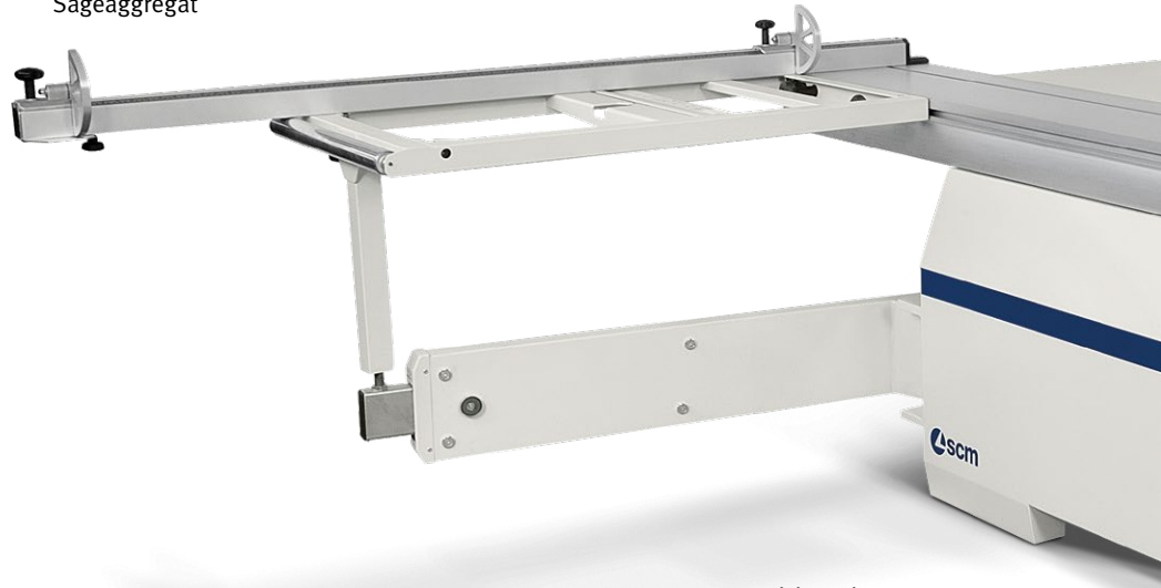
minimax si x 32 A 3 UP zeigt Option „2 Sägeblattgeschwindigkeiten“
