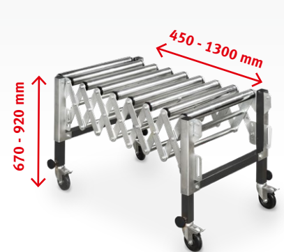
SRB 130 Scherenrollenbahn Höhe einstellbar, Rollenlänge 480 mm
