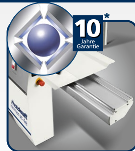
Aluminium-Schiebeschlitten ► Schiebeschlitten wird durch tausendfach bewährtes Kugelkontaktsystem hochpräzise und leichtgängig geführt ► Zehn Jahre HOLZKRAFT-Garantie* auf Verschleiß der gehärteten Führungsbahnen
