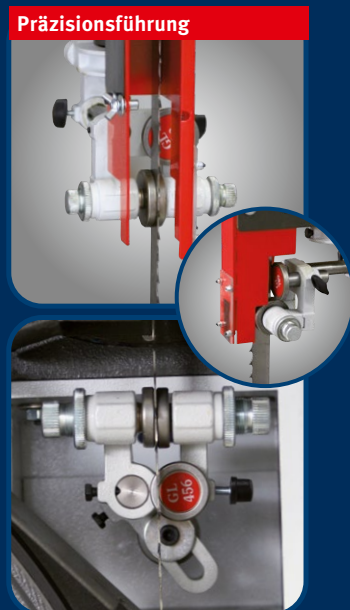
Präzisions-3-Rollen-Sägebandführung mit Führungsrollen oben und unten und Feineinstellung
