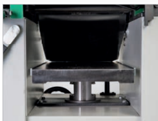
Dicketischverstellung über Handrad, Skala und numerischer Anzeige
