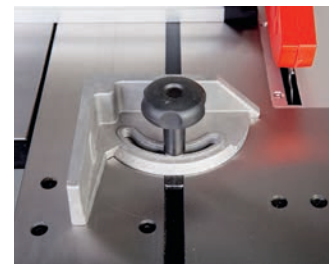
Stufenlos verstellbarer Winkelanschlag von -45° bis +45°
